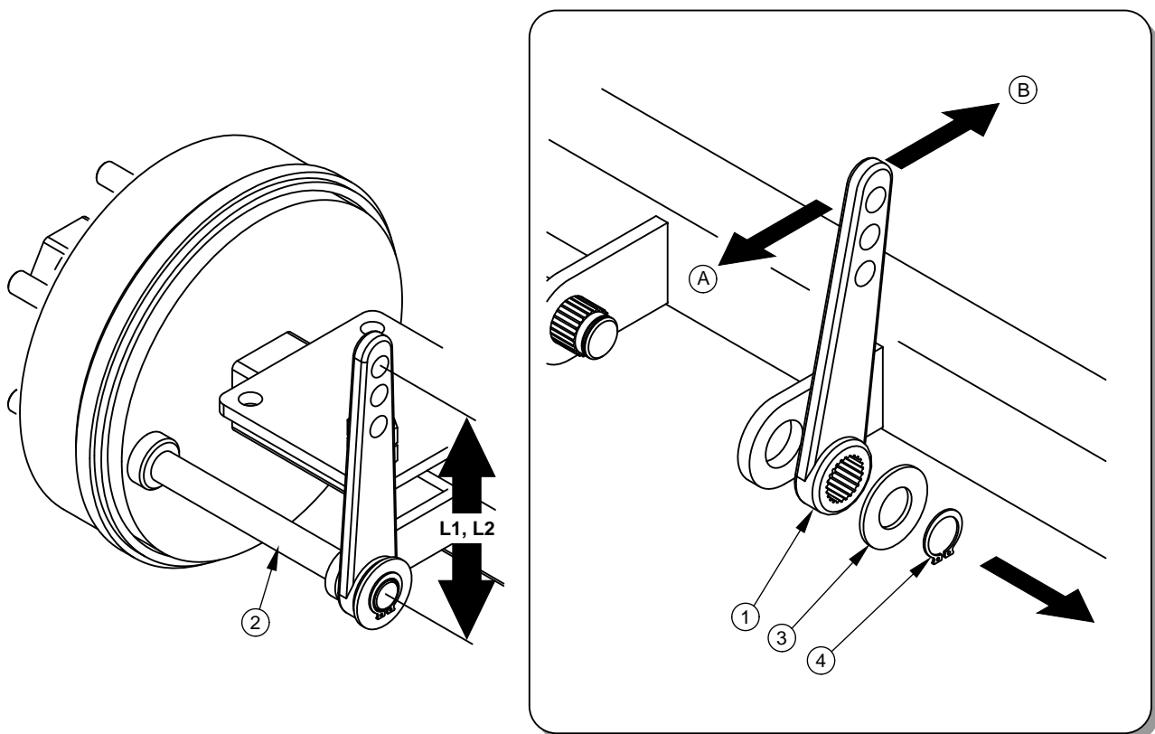
RYСУNEK 5.4 Regulacja hamulców mechanicznych osi jezdnych
