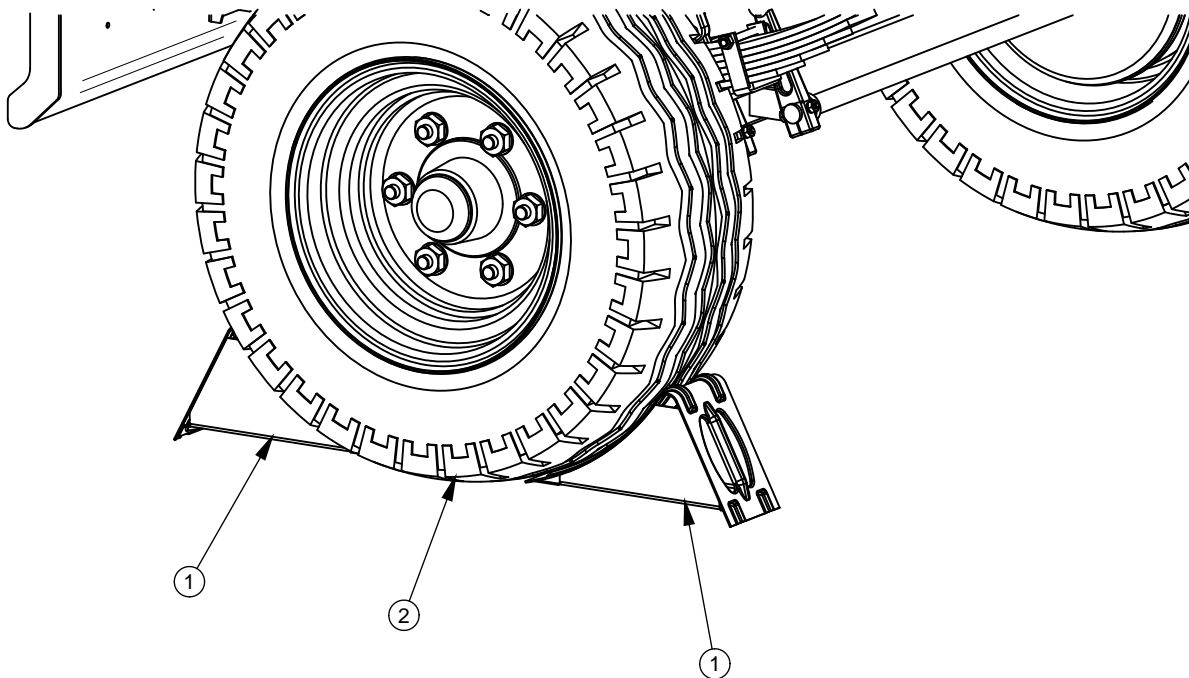
RYSUNEK 2.1 Sposób ustawiania klinów
